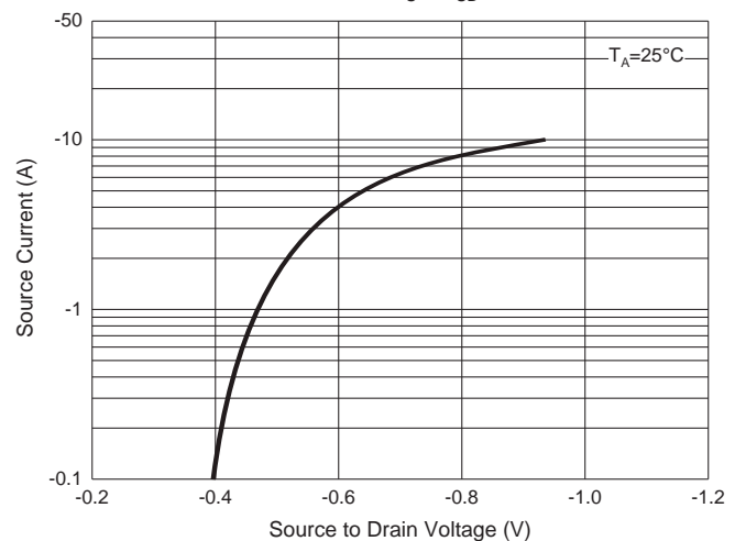
Fig. 6 - I_S — V_{SD}
