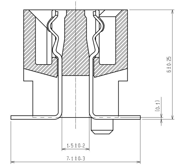
A-A (10:1)
