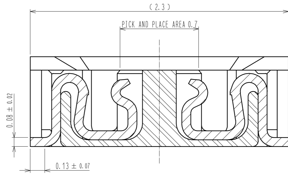
A-A(50:1)
