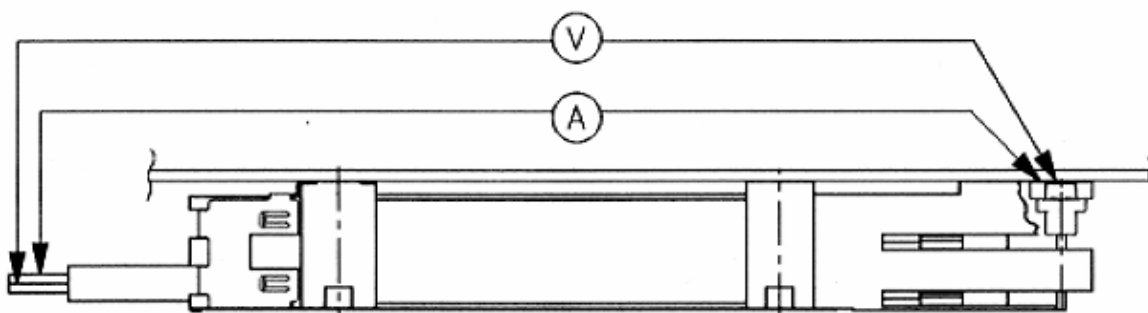
Fig.5 ローレベル総合抵抗測定図
