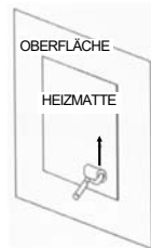
Abbildung 3: Aufrollen der Heizmatte
