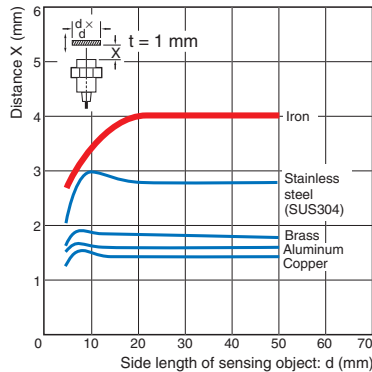
E2E-X4MD□
