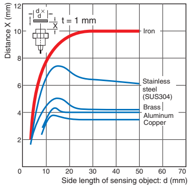
E2E-X10D□/-X10T1
