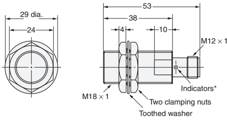
Diagram 20 E2E-X7D□-M1(G)/E2E-X5E□-M1/X5F□-M1 E2E-X5Y□-M1
