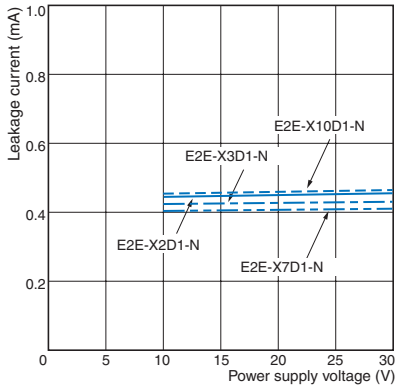
E2E-X□D□
