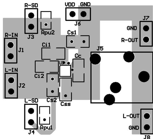
Bottom Layer
