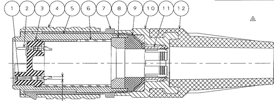
断面 A-A
