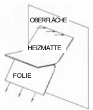
Abbildung A: Entfernen der Folie
