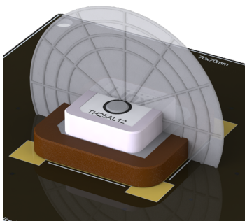
XZ-Plane Gain
