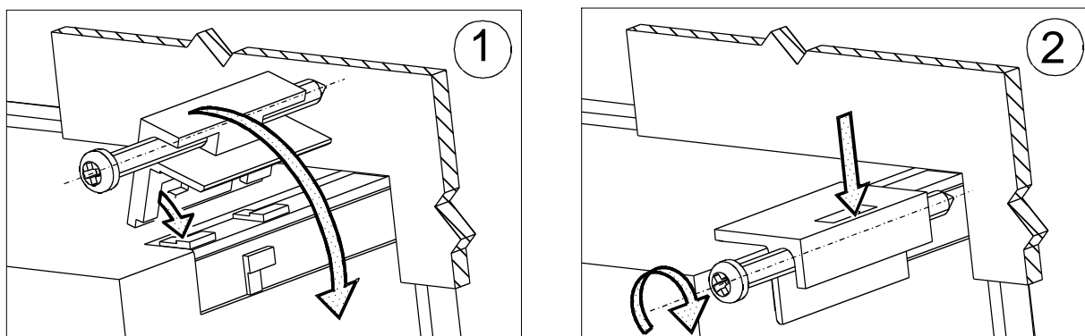
Fig. 2. Meter fitting
