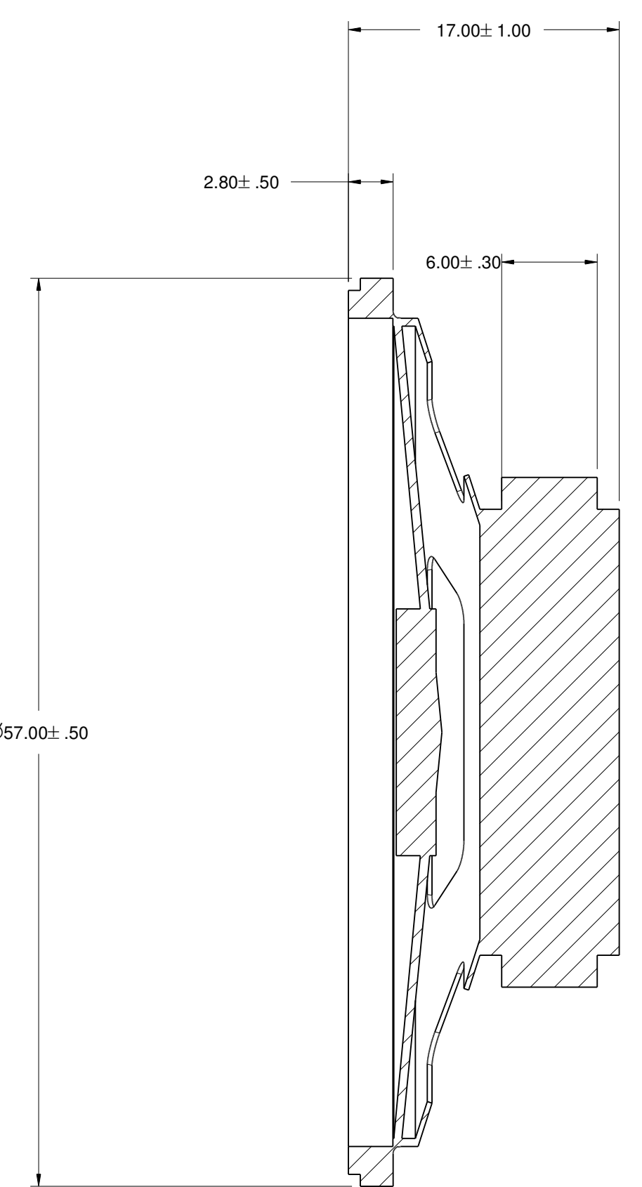
Section A-A
