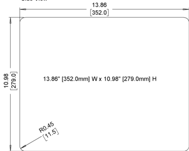
Cutout Dimensions
