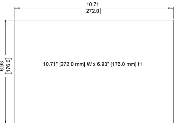
Cutout Dimensions
