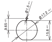
〈パネル取付け孔寸法図 Panel cut-out dimensions〉
