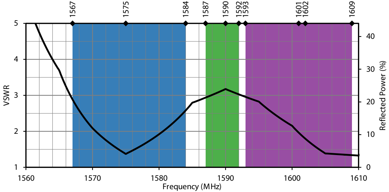
Figure 2. GNSSCP-TH18L1 VSWR
