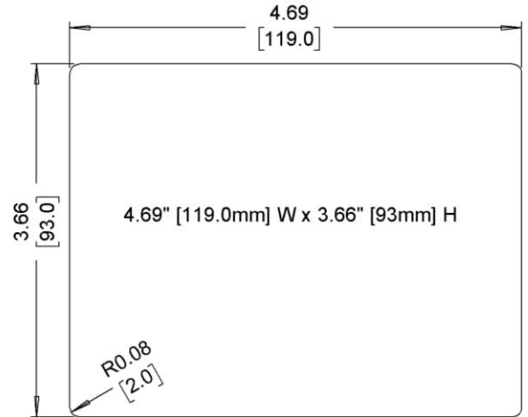
Cutout Dimensions
