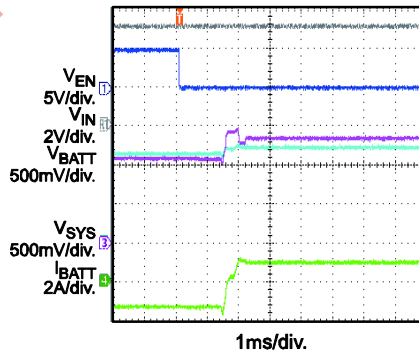
En On V_{BATT} = 3.7V , I_{SYS} = 1.5A ( V_{BATT} & V_{SYS} has 2.5V Offset)
