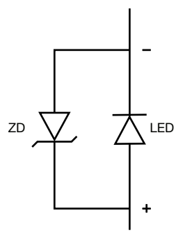
Fig. 9 - Wiring Diagram
