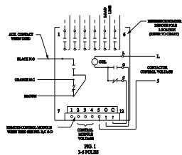
FIG. 1 24 POLES
