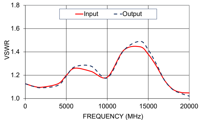
EQY-5-24+ VSWR
