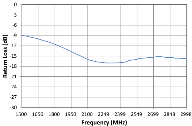
Lo port Return Loss
