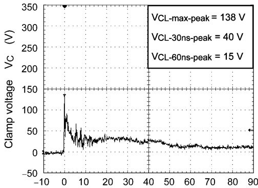
Fig. 6.1.3 +15 kV
