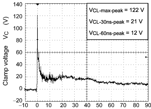
Fig. 6.1.1 +8 kV
