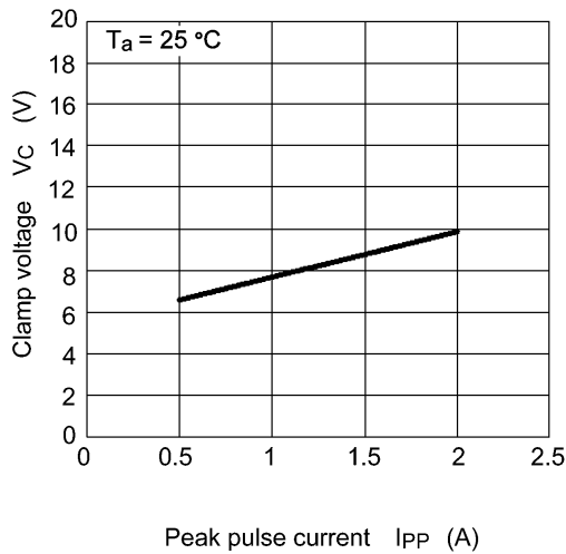
Fig. 6.3.1 V_C - I_{PP}
