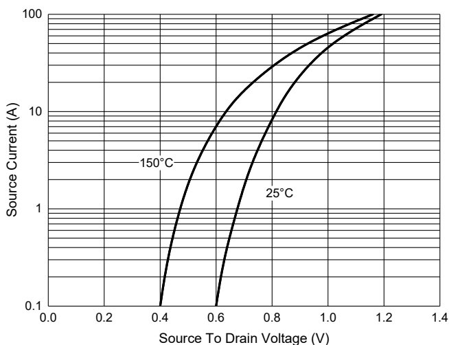
Fig. 6 - I_S - V_{SD}
