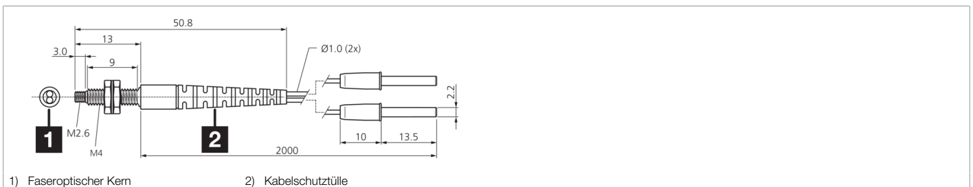
1) Faseroptischer Kern 2) Kabelschutztülle
