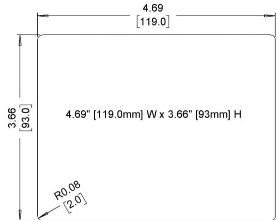
Cutout Dimensions
